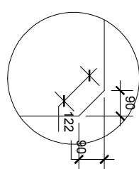
szczegół A
